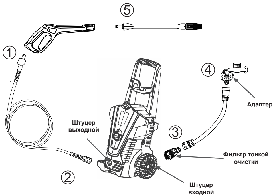
Рис. 2 Сборка аппарата
