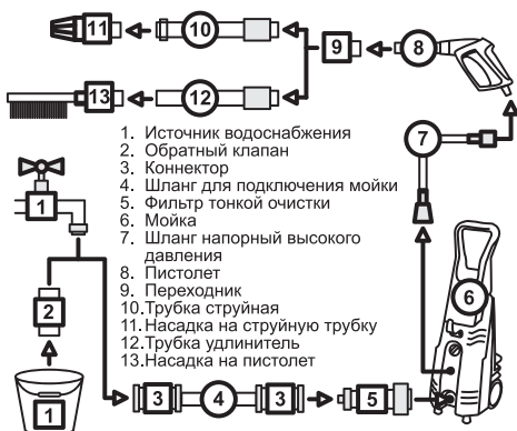
Рис. 13 Схема подключения аппарата с дополнительным оборудованием
