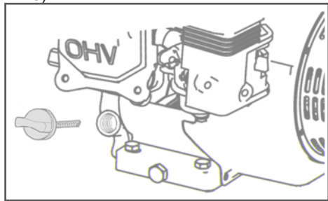
Рис. 5 Крышка-щуп маслосазливной горловины
