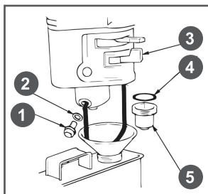
Рис. 18 Обслуживание фильтра-отстойника
