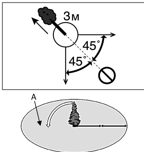
Рис.12 Зона безопасности при валке дерева
