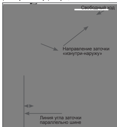
Рис. 18 Определение угла заточки
