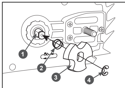
Рис. 24 Снятие ведущей звездочки
