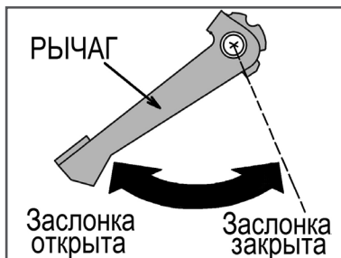
Рис. 9 Рычаг управления воздушной заслонкой (вид сверху)
