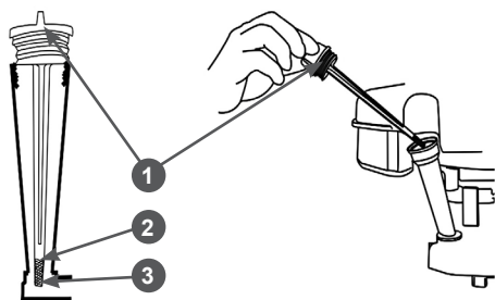
Рис. 22 Крышка-щуп маслозаливной горловины
