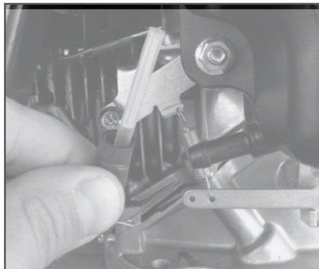
Рис. 12 Топливный фильтр
